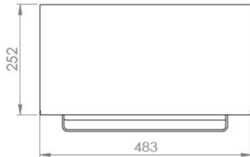
TO3
